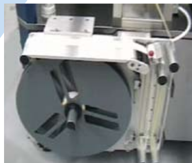
Presvolgitoro motorizzato PR06 Powered unwind unit PR06 Porte-bobine motorisé PR06
